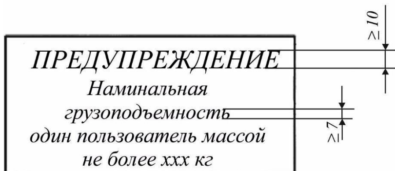
Рисунок 15 - Образец стандартной надписи с информацией о грузоподъемности
