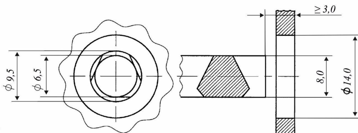
Рисунок 9 - Треугольный ключ для запираания двери
