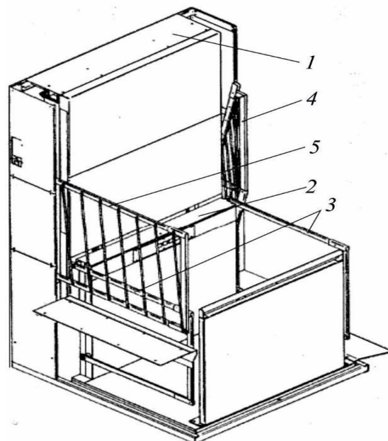
Рисунок 12 - Подъемная платформа с ограждением входных проемов шлагбаумами
