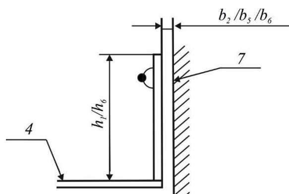
г) Ограничение доступа к краям платформы; предохранительный неперфорированный барьер для платформы с перемещением более 2000 мм, использование барьера в качестве поручня
