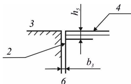
а) Вход на верхнюю или промежуточную посадочную площадку, фартук
