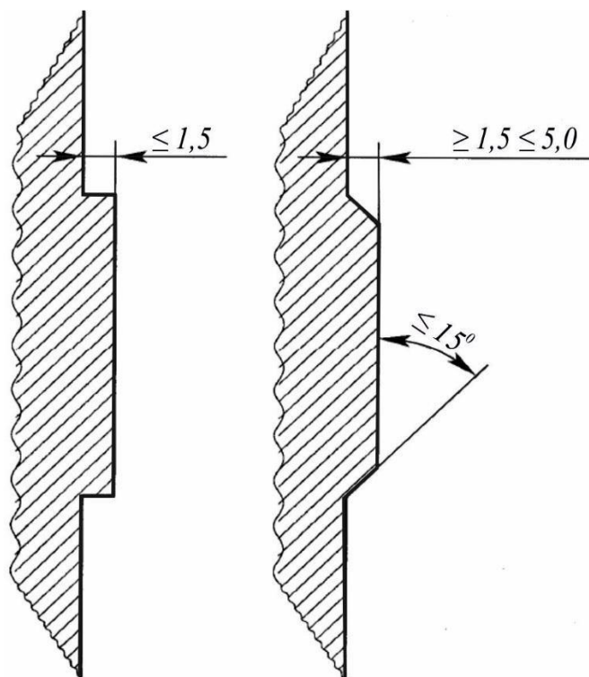
Рисунок 11 – Размеры допустимых выступов в зонах перемещения
